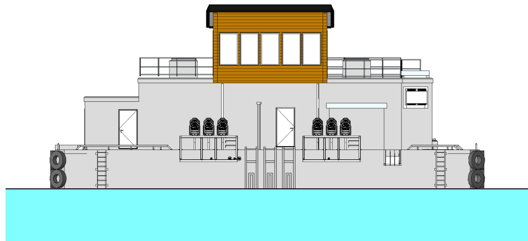
2 FASADE MOT MÆRDER 1 : 200
